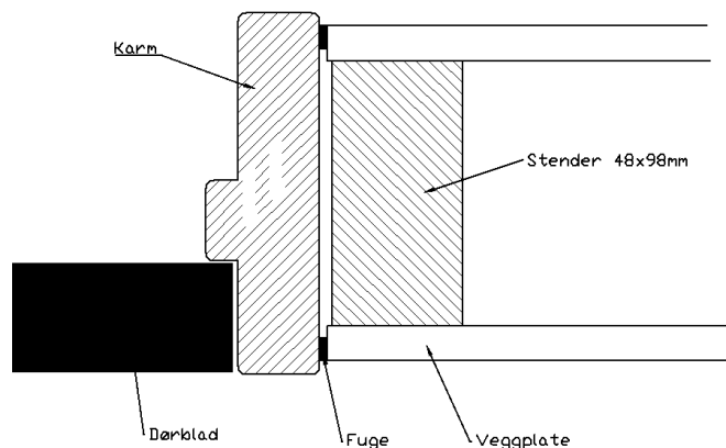
Skisse som viser hvordan karmen monteres i veggen.
