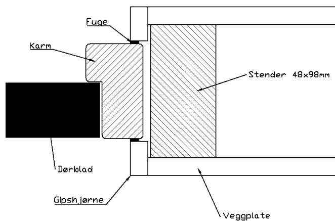
Skisse som viser hvordan karmen monteres i veggen.
