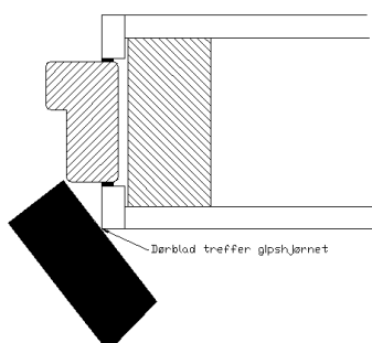
Detalj av monteringen. Her er det brukt gipshjørne. Gulvlisten er gjæret og avsluttes inn mot karmen. Hengsle Tectus 340 3D. Denne døren er malt med ulike hvitnyanser på hver side.
